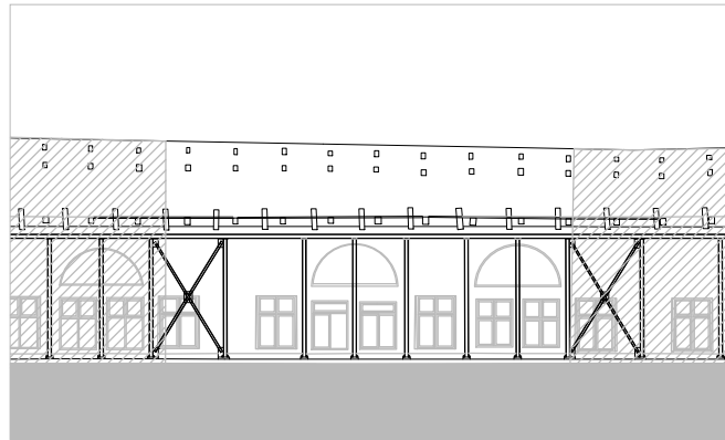
LONG SECTION A-A'
